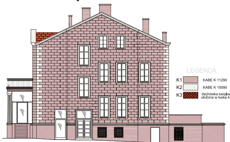
elewacja zachodnia
